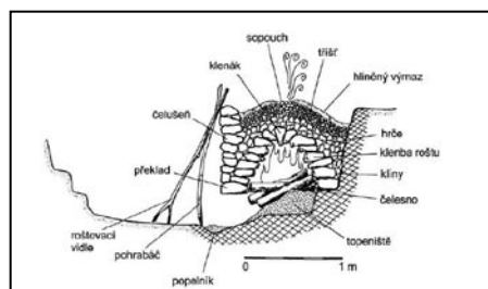
Mokrý – Spálená seč. Orientační podélný řez experimentální vápenickou pecí postavenou podle nálezu zbytků pece ze šestnáctého století. Autor kresby Petr Kos.
