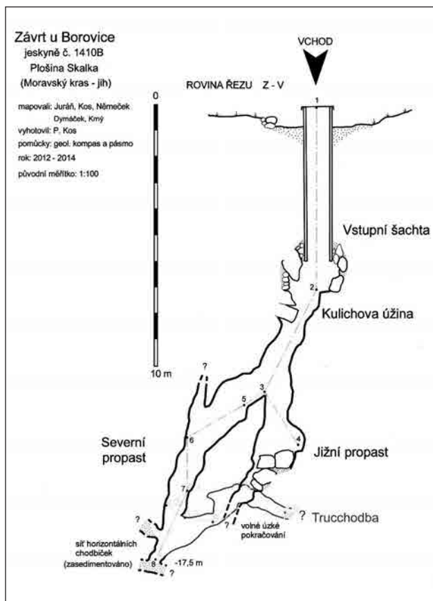
Závrt u borovice – bokorys
