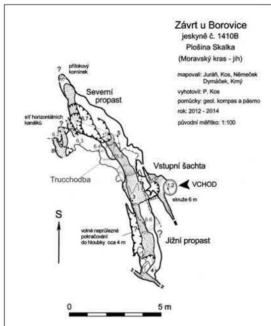
Závrt u borovice – půdorys
