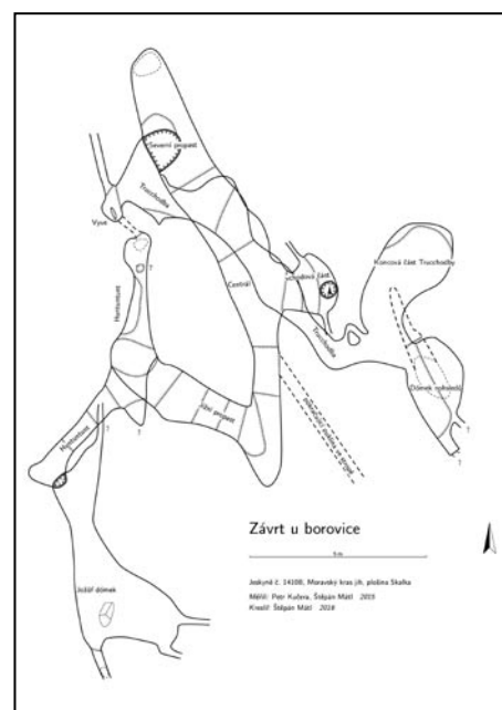
Nákres půdorysu Závrtu u borovice.
